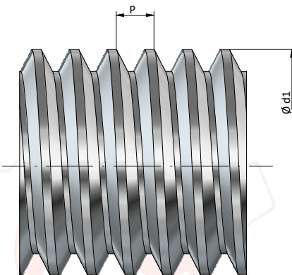
Husillo rosca trapecial S/DIN 103- 1 entrada. Material : C - 45
